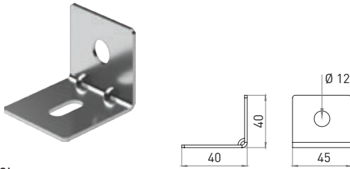
Tijli Kanal Taşıyıcı Cable Tray Carrier (Threaded Rod For)
