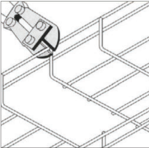
Yan Kenar Üst Telleri Kes Side Edge Upper Wires Cut
