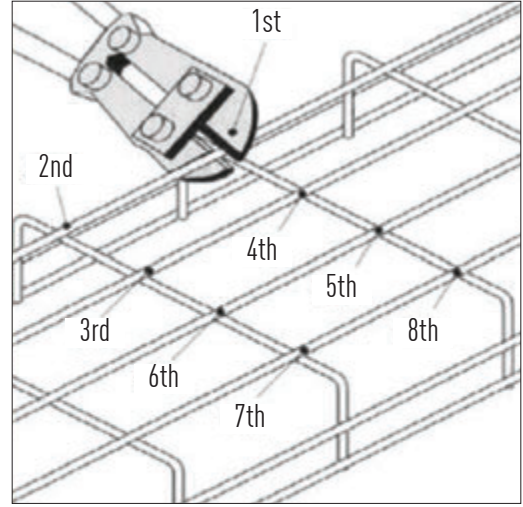
Kesme Sıralaması Cutting Order
