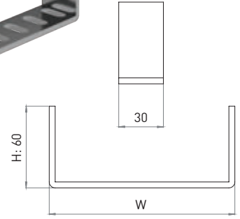
Deliksiz Uzun U Askı Ayağı Non Perforated U Long Bracket
