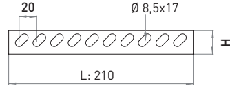
Kanal Separatörü Cable Separator
