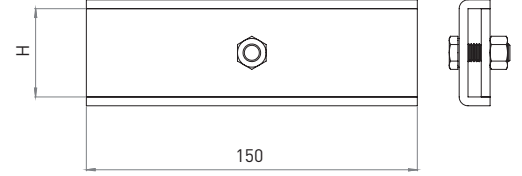
Gemi Tipi Kablo Merdiveni Ek Parçası Marine Type Cable Ladders Straight Connectors
