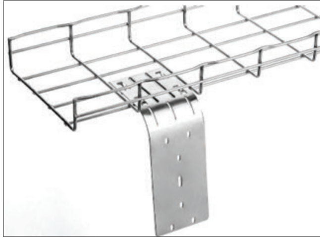
Kanal Taşıyıcı Tray Carriers
