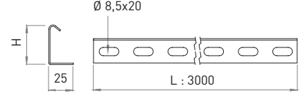
Kanal Separatörü Cable Separator
