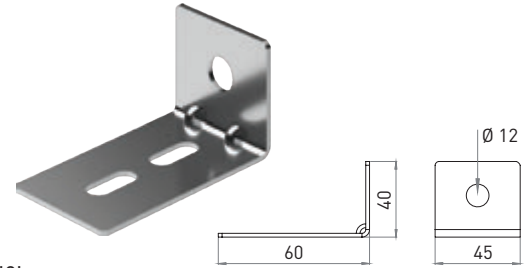
Tijli Kanal Taşıyıcı Cable Tray Carrier (Threaded Rod For)
