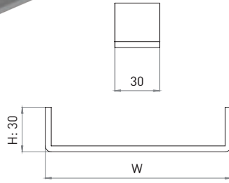
Deliksiz Uzun U Askı Ayağı Non Perforated U Long Bracket
